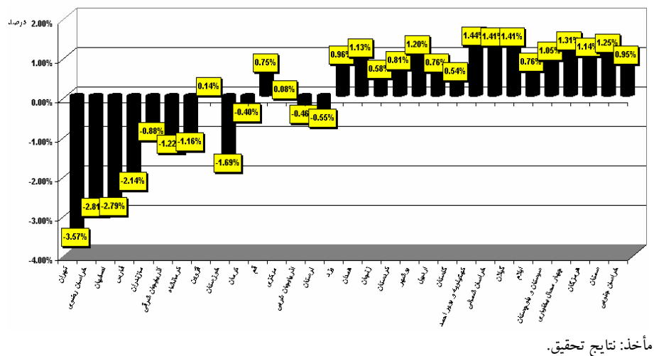
نمودار ۳. تعدیل در درصدهای سرمایه‌گذاری بر اساس شرایط ریسک و عدم قطعیت
