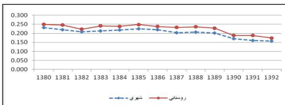
نمودار ۴. مقایسه توزیع درآمد شهری و روستایی بر اساس شاخص اتکینسون \epsilon = 0.9
