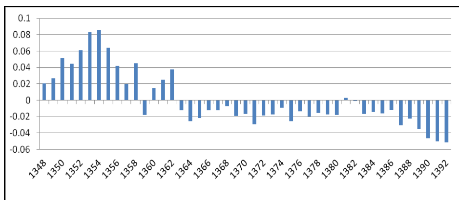
نمودار ۳. روند انحراف از میانگین ضریب جینی کشور در فاصله سال‌های ۹۲-۱۳۴۸ ش
